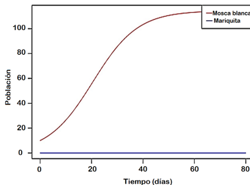
Figura 1. Crecimiento poblacional de la mosca blanca en ausencia de depredadores.
