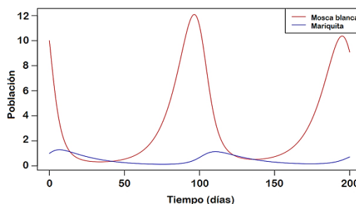
Figura 2. Crecimiento poblacional de la mosca blanca con presencia de la mariquita y el control óptimo.
