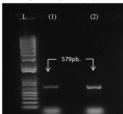
Figura 2. Productos PCR amplificados utilizando el juego de primers F1 y R1 para ambos carriles (1) y (2). Accesoión: PER018279 y PER018283 para los carriles (1) y (2) respectivamente.
