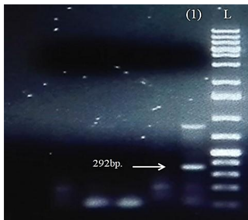
Figura 4. Productos de la PCR-anclada visualizados en gel de agarosa. El carril (1) corresponde al fragmento de tamaño 292bp de la región no codificante 3' del ARNm de la probable 1-FEH de yacón.
