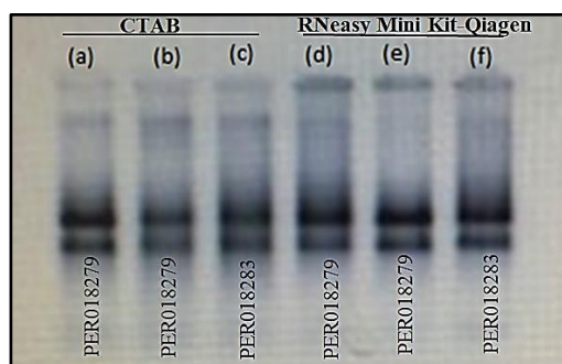
Figura 1. Extracción de ARN total mediante los protocolos CTAB [(a), (b), (c)] y RNeasy Mini Kit-Qiagen [(d), (e), (f)]. Accesoión: PER018279 [(a), (b), (d), (e)], PER018283 [(c), (f)].
