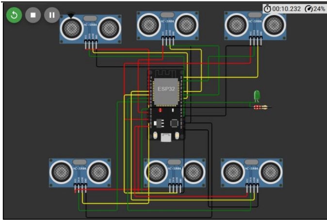
Fig. 1. Simulación del circuito ESP32 con sensores HC-SR04 en Wokwi.
